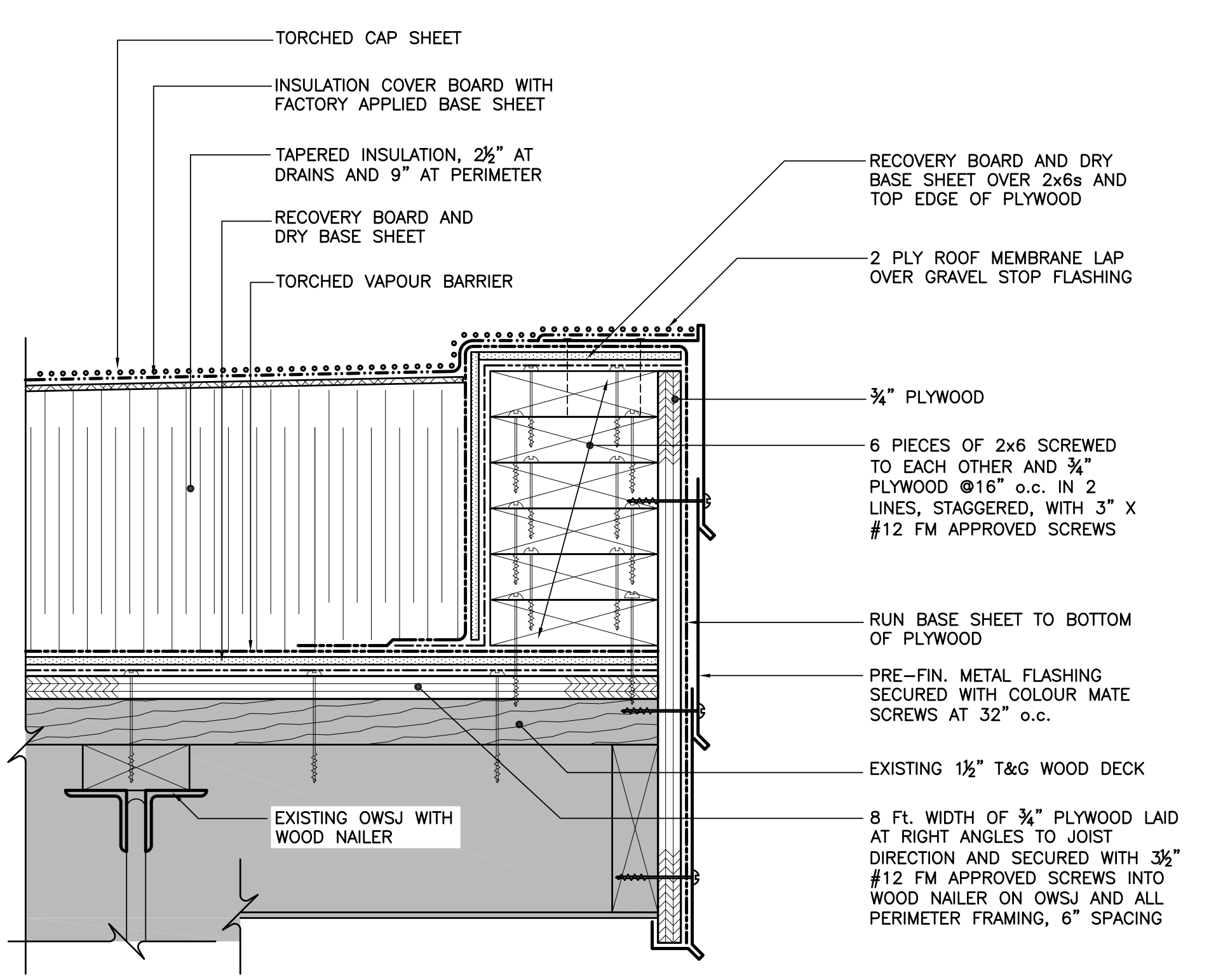
3 A-1 PARAPET DETAIL SCALE: 3" = 1'-0"
