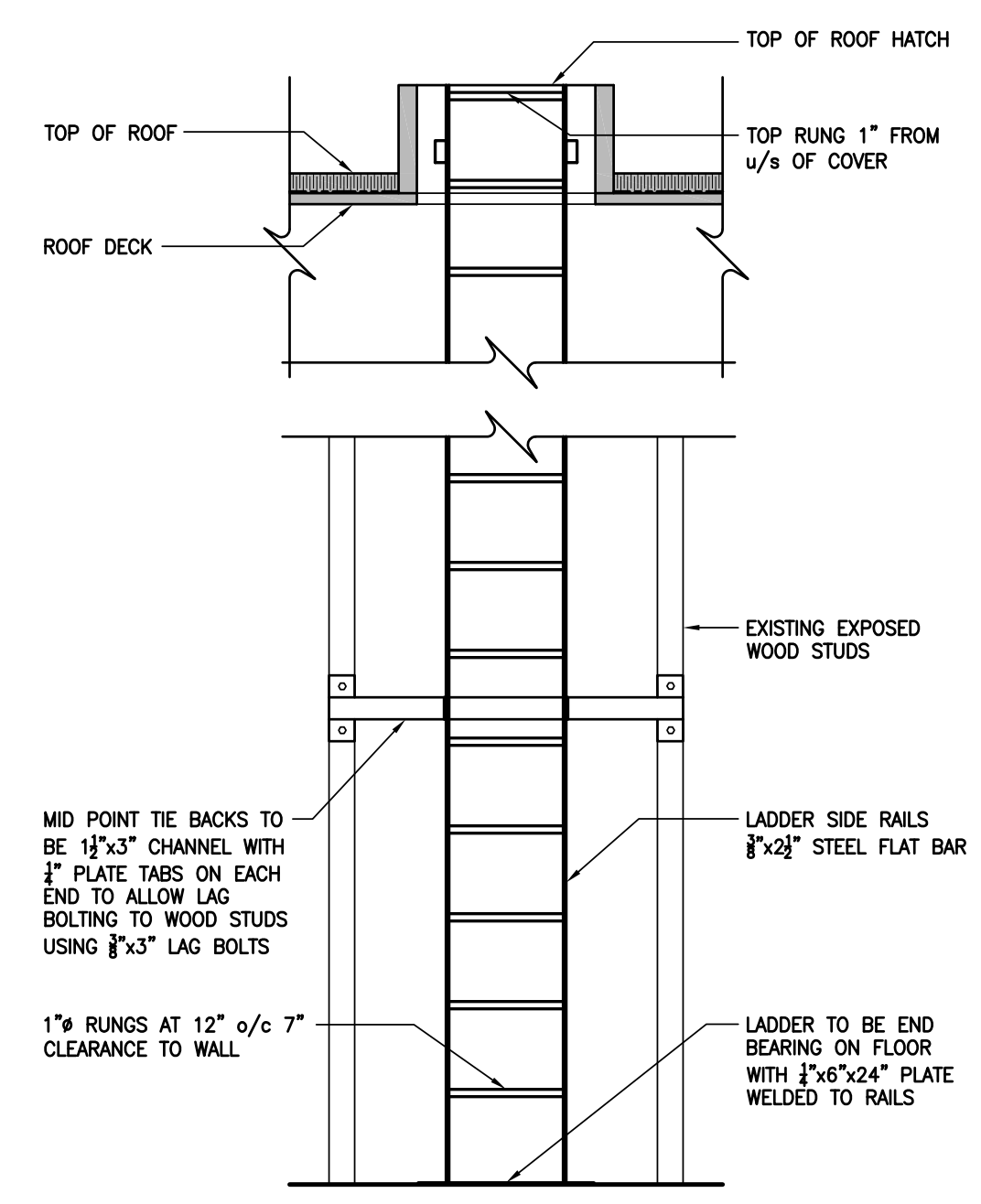
6 A-1 ELEVATION - ACCESS LADDER SCALE: 1/2" = 1'-0"
