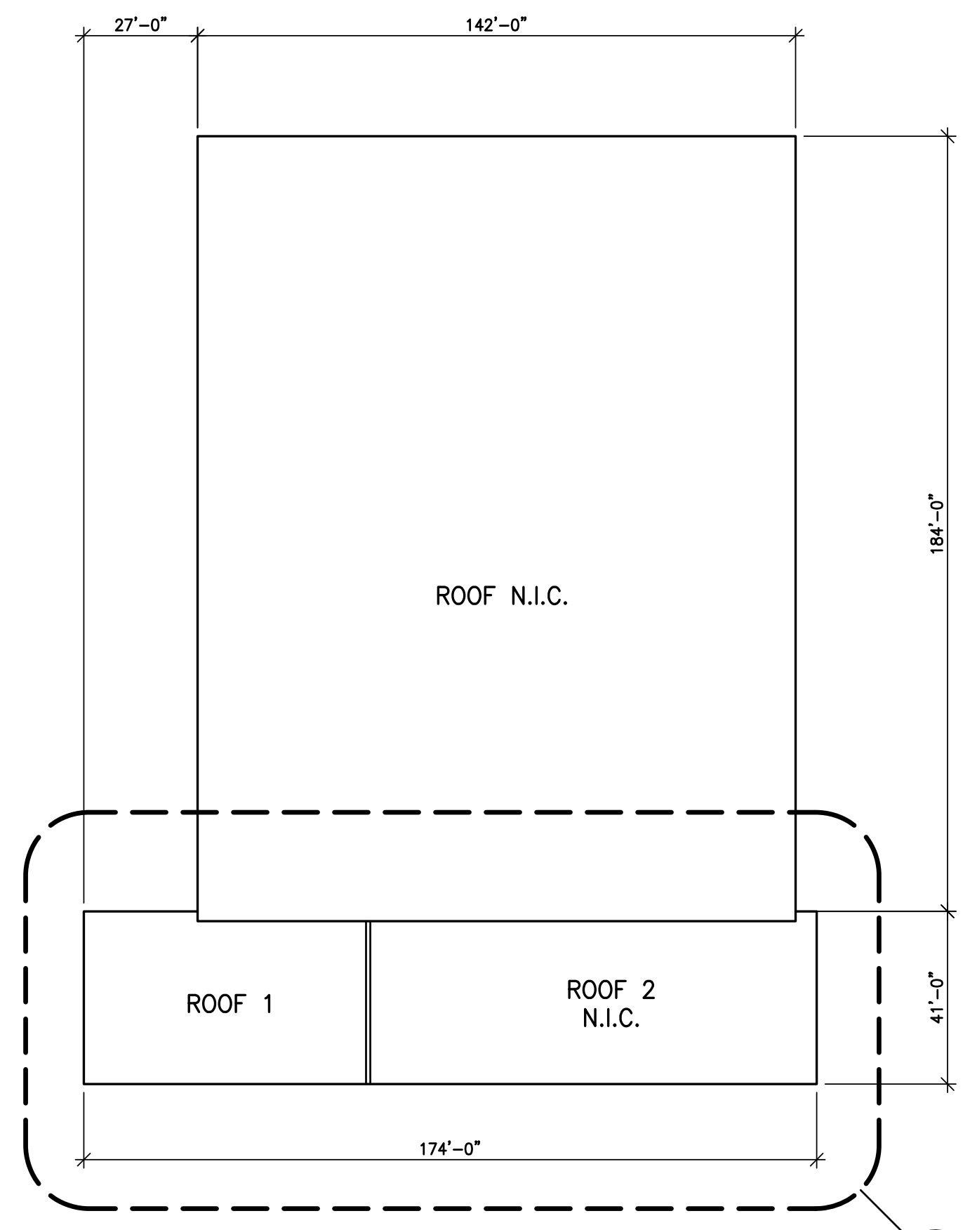
1 A-1 KEY PLAN SCALE: 1/32" = 1'-0"
