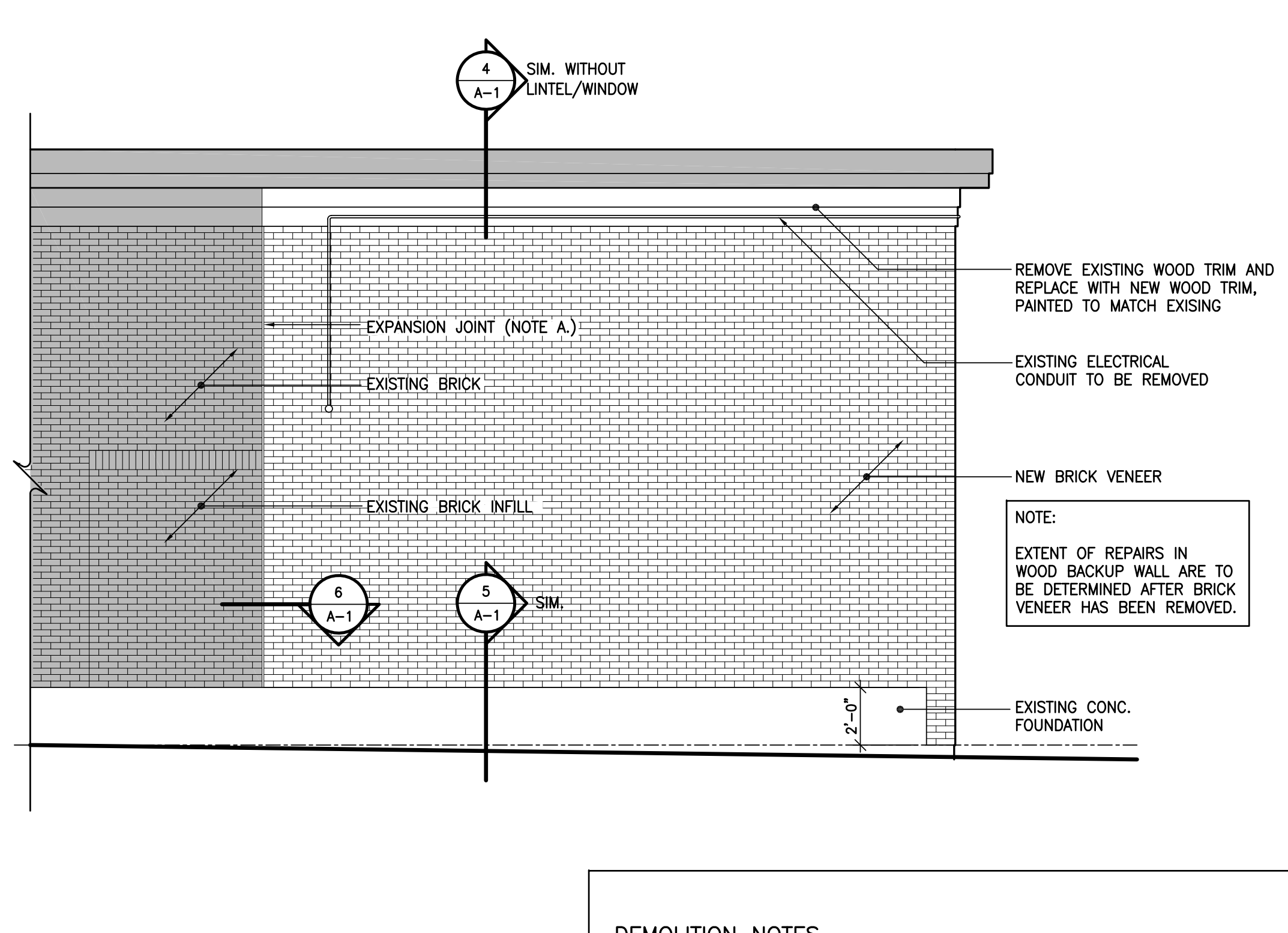
3 A-1 EAST ELEVATION SCALE: 1/4" = 1'-0"
