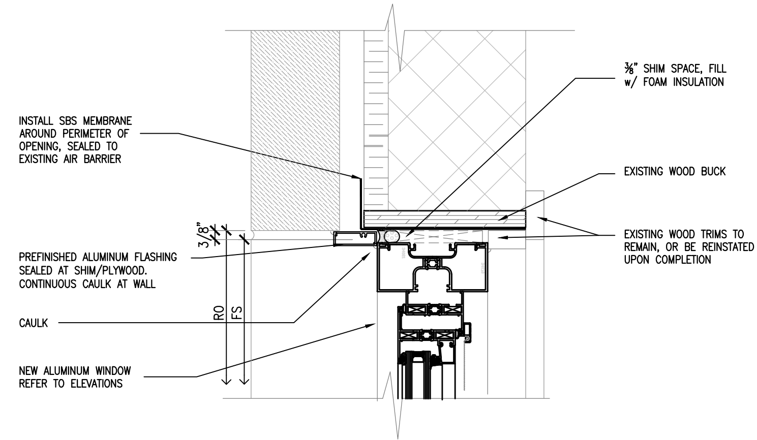
3"=1'-0" D1 SECTION - WINDOW JAMB A-301
