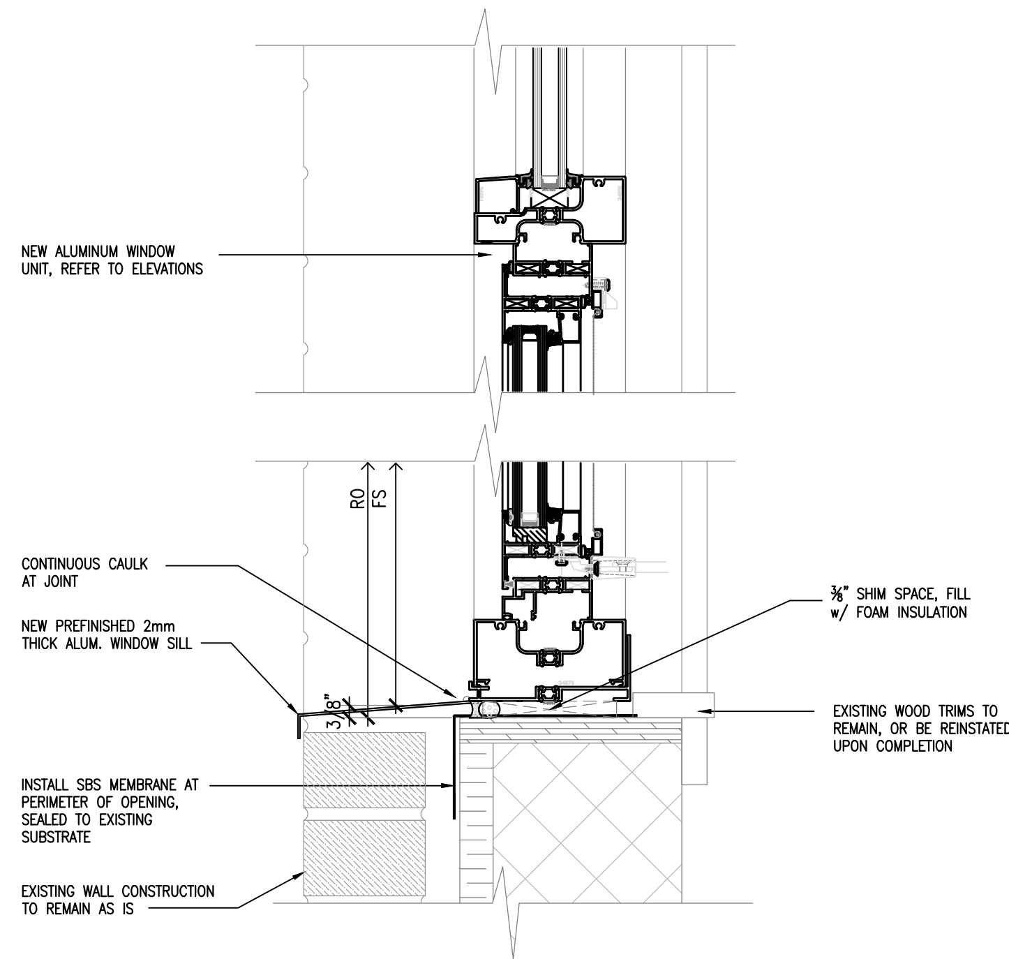
3"=1'-0" D2 SECTION - WINDOW SILL A-301
