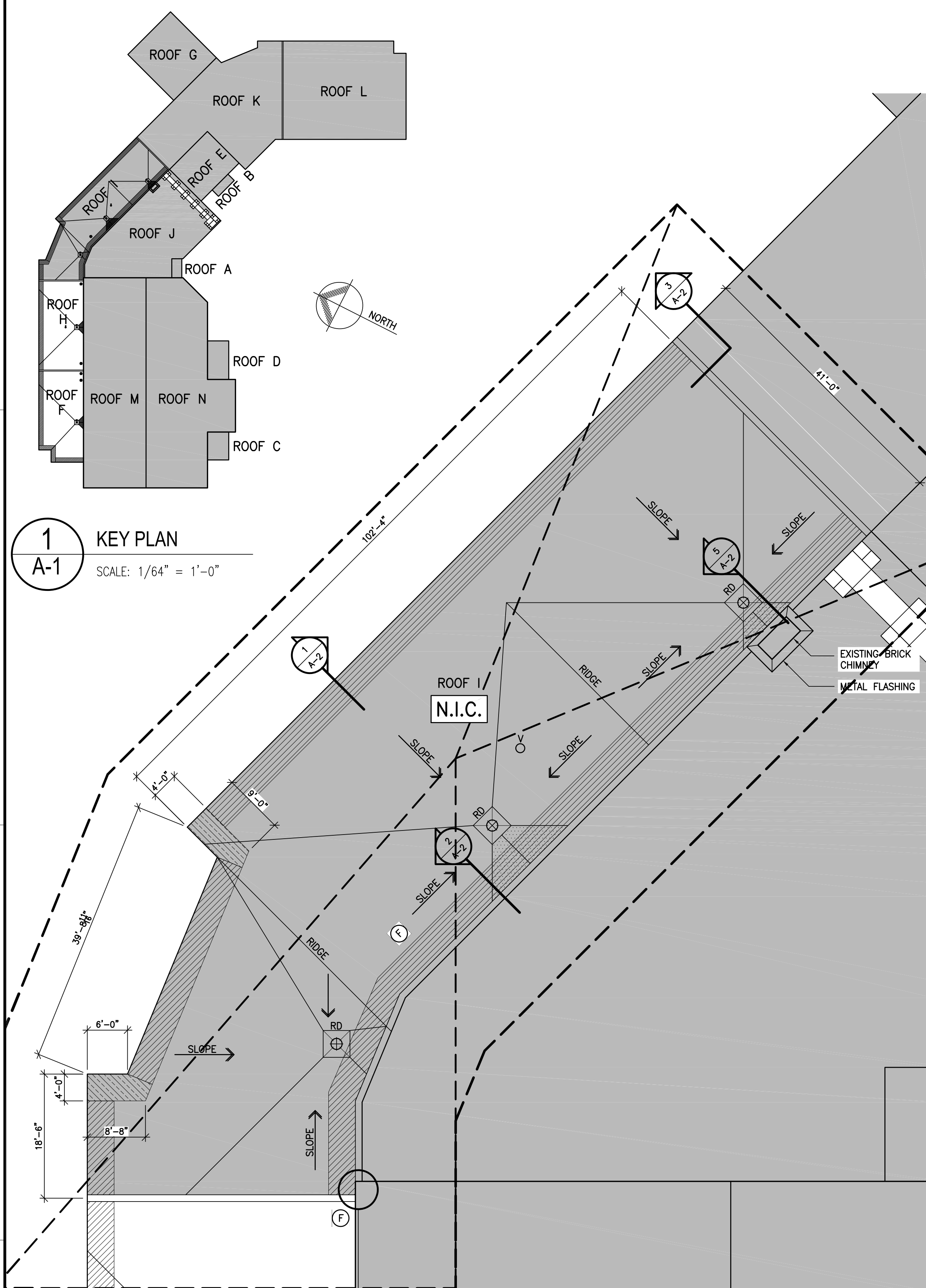
2 PLAN - ROOF 'I' N.I.C. A-1 SCALE: 3/32" = 1'-0"
