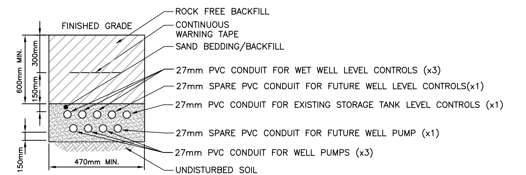
SECTION 1 SCALE: N.T.S.
