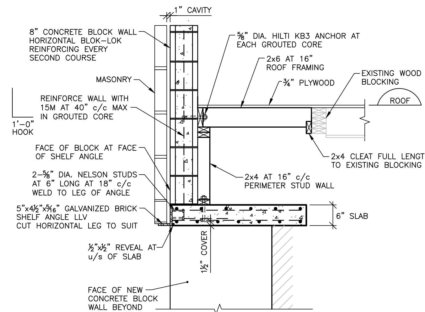
101 SECTION SCALE: 3/4"=1'-0"
