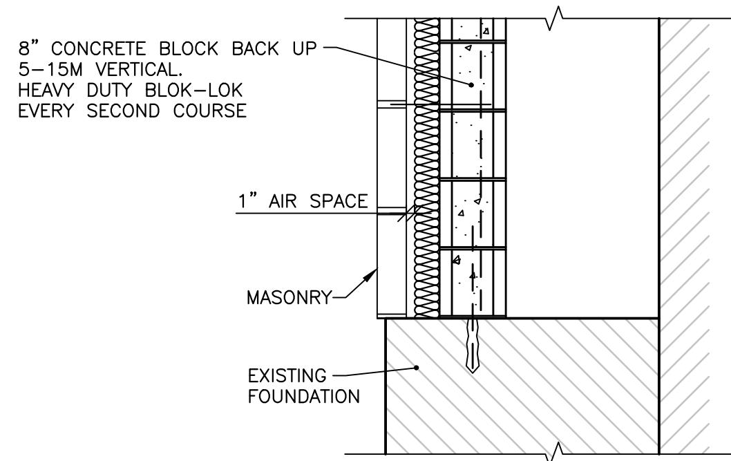
100 SECTION SCALE: 3/4"=1'-0"
