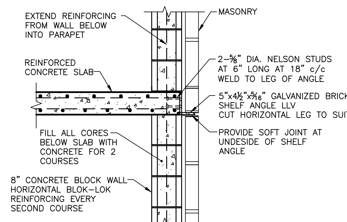
102 SECTION SCALE: 3/4"=1'-0"
